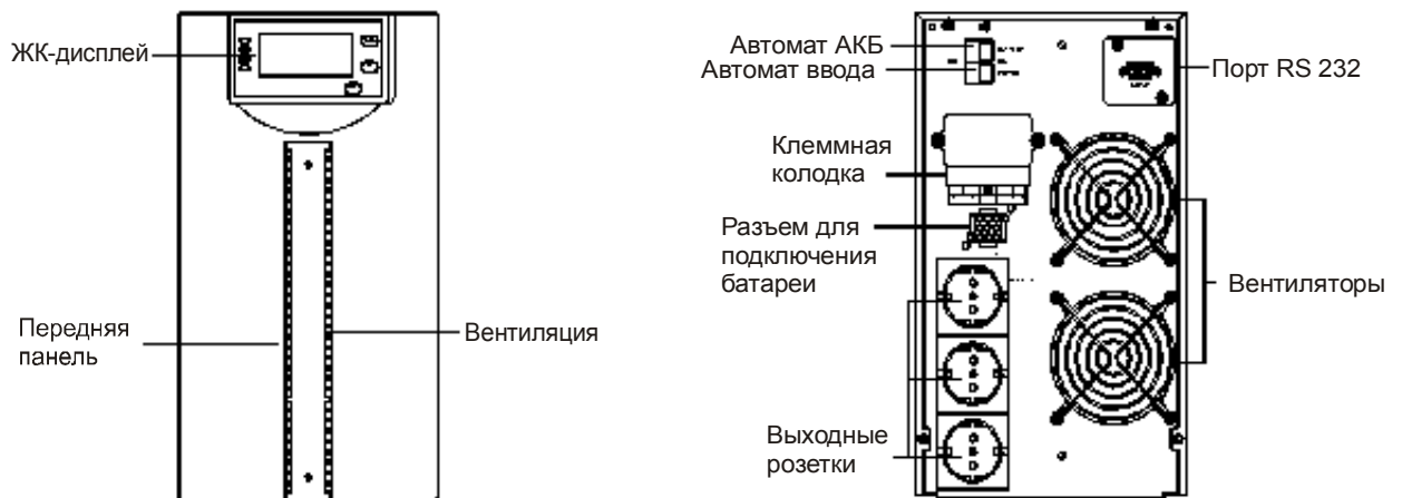
Рис. 2-3 Передняя и задняя панель KR2000LCD и KR3000LCD
