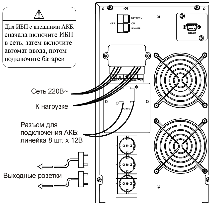
Рис. 3-3. Схема подключения KR2000LCDL, KR3000LCDL
