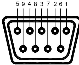
Рис. 2-4. Распайка разъема RS232
